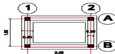
latrine à 02 compartiments FONDATION
