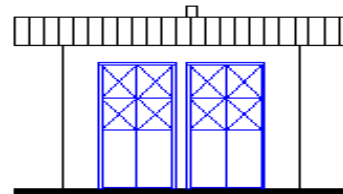
latrine à 02 compartiments FACADE PRINCIPALE
