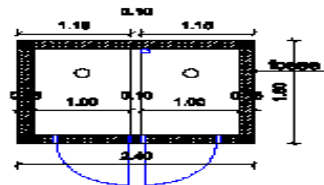
latrine à 02 compartiments DISTRIBUTION
