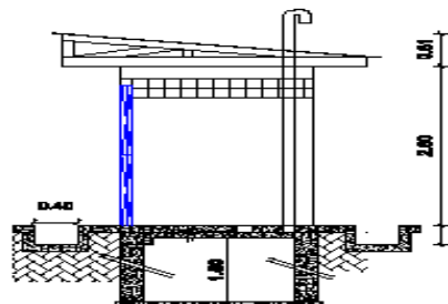
latrine à 02 compartiments COUPE
